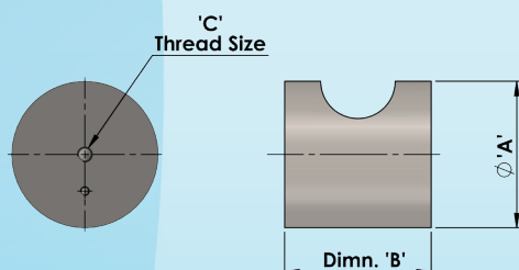
CCDK CYLINDER c/w SCALLOP CENTRE DOOR KNOB
