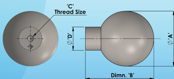
BCDK BALL SHAPE CENTRE DOOR KNOB
